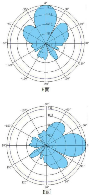
信号方向图
