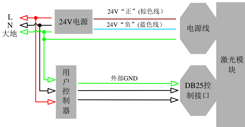
图 4 电气连接图
