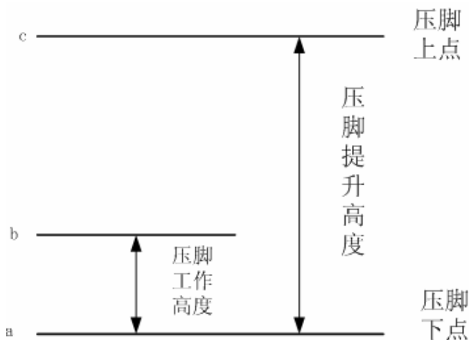
压脚提升示意图
